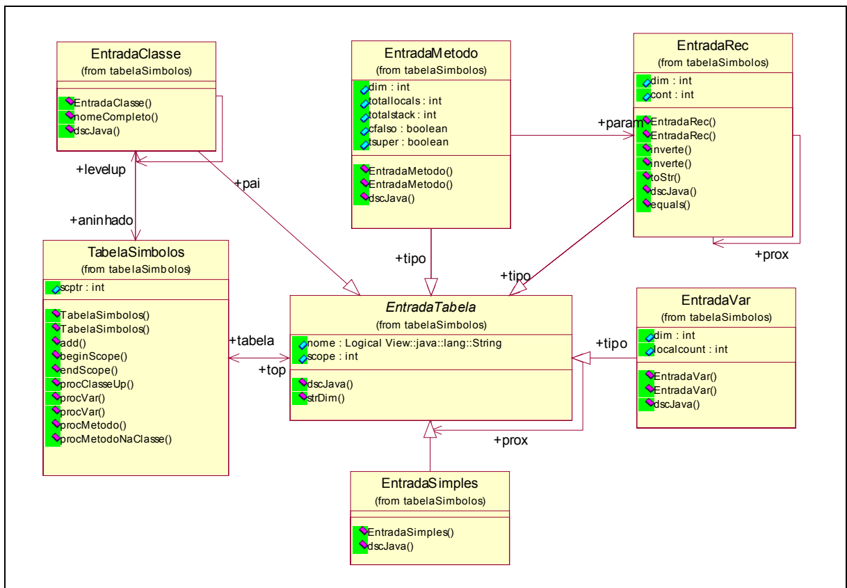
Figura 33 - Diagrama de classes do pacote tabelaSimbolos
