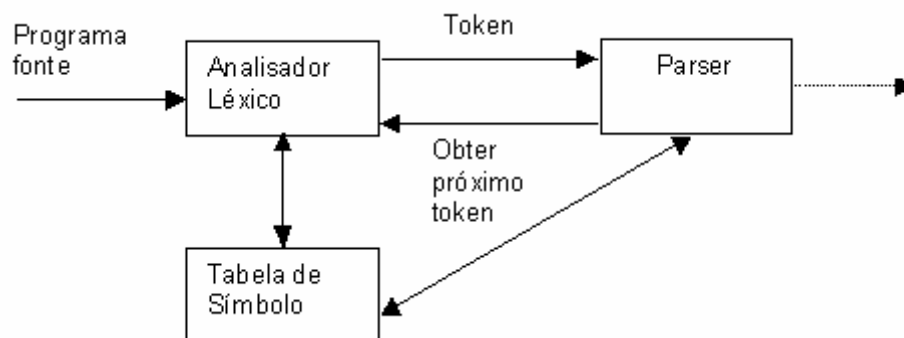
Figura 3 - Analisador Léxico
